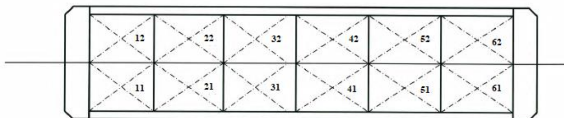
Рисунок 2 – Схематичное расположение танков на палубе нефтеналивной баржи HC-1001
