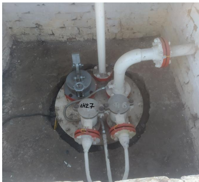
Рисунок 1 – Общий вид резервуара РГС-10
