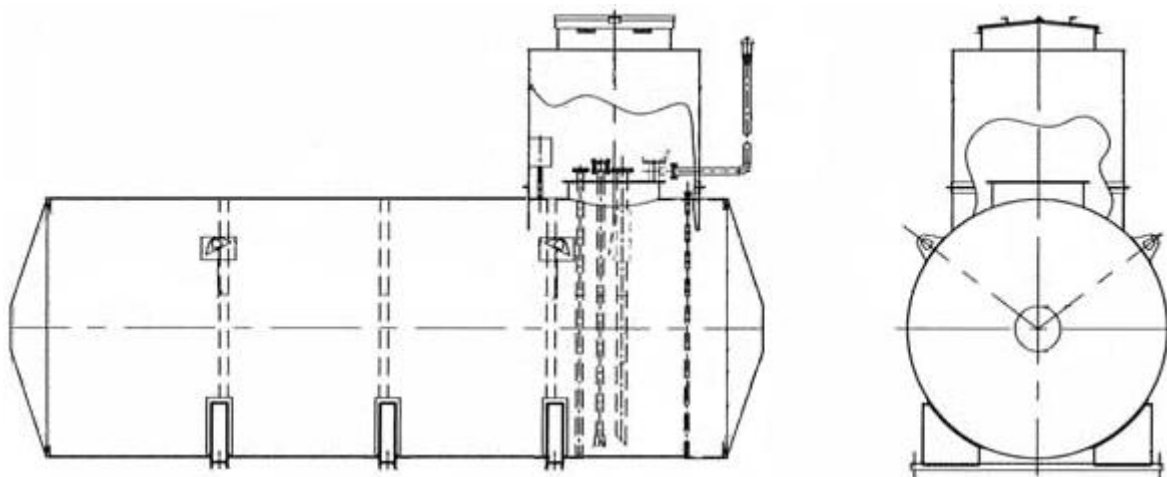
Рисунок 3 – Общий вид резервуаров PGC-25
