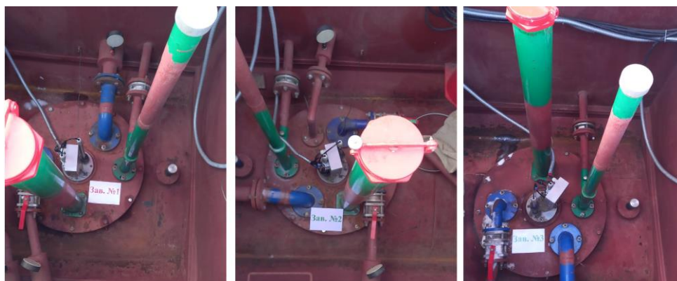
Рисунок 1 – Общий вид резервуаров РГС-25
