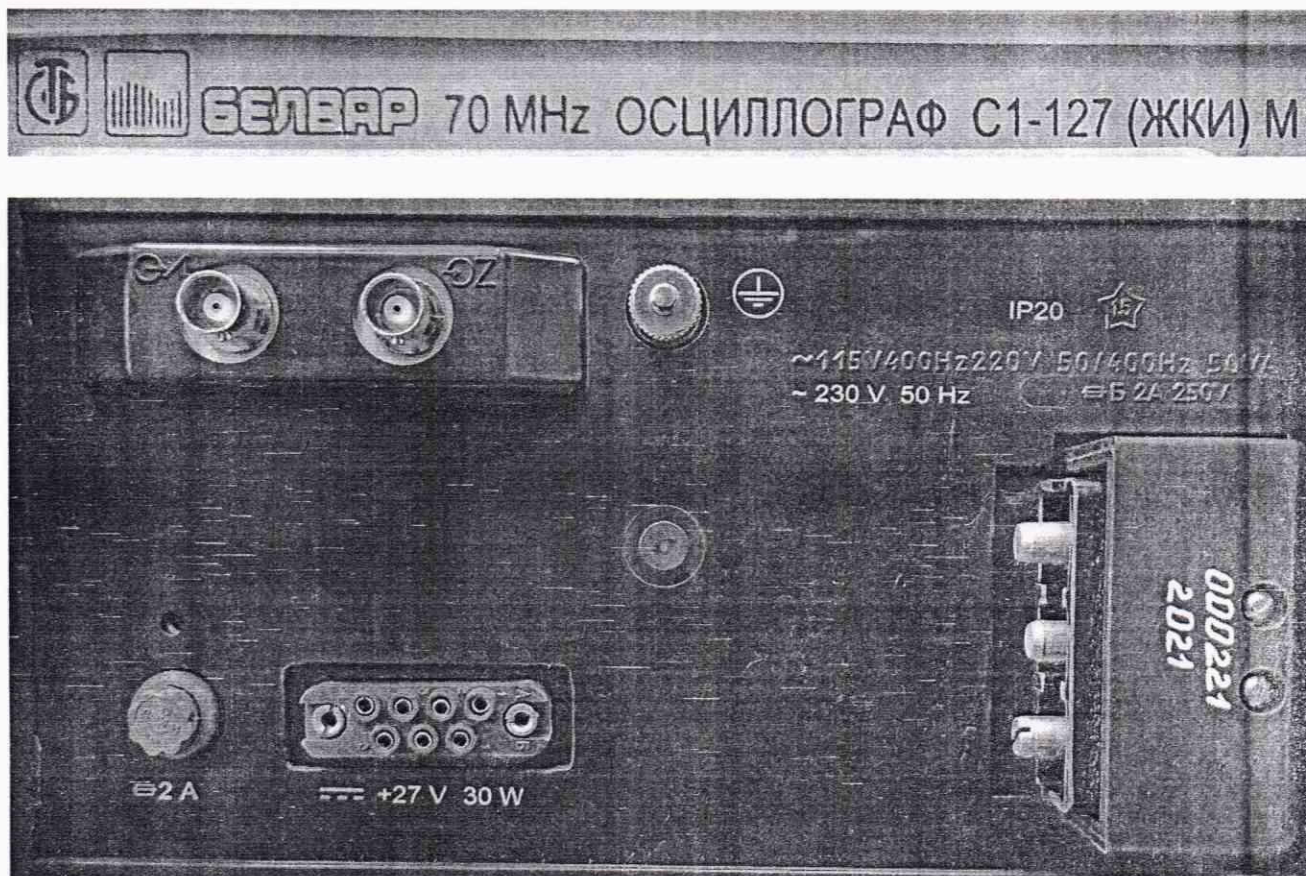
Рисунок 1.2 – Маркировка осциллографа
