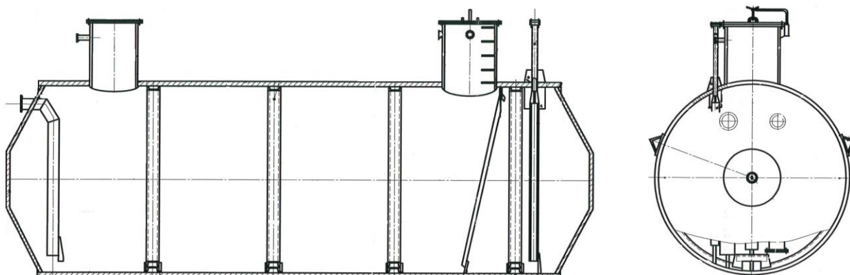
Рисунок 2 – Общий вид резервуара РГС-50 Пломбирование резервуара РГС-50 не предусмотрено.
