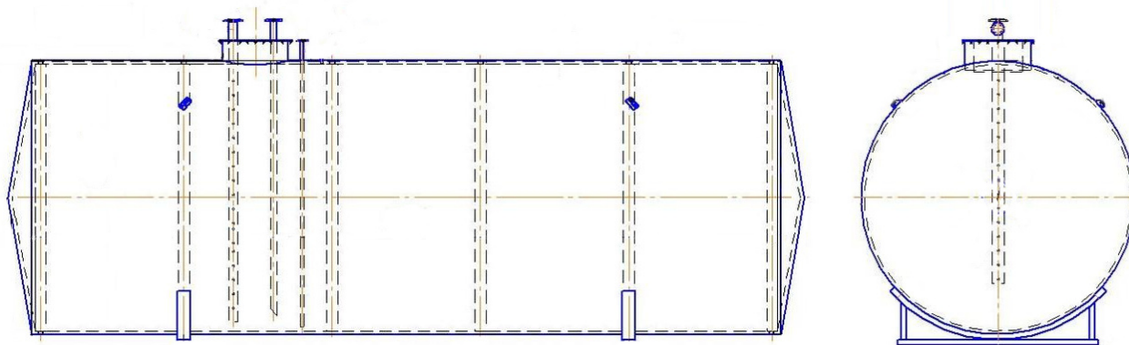
Рисунок 5 – Общий вид резервуаров РГС-25
