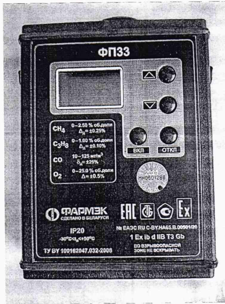
Рисунок 1.1 – Внешний вид газоанализатора
