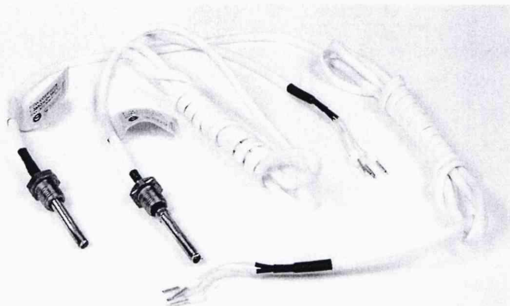
Рисунок 1.1 – Фотография общего вида комплекта ТСПА-К исполнения PL (носит иллюстративный характер)
