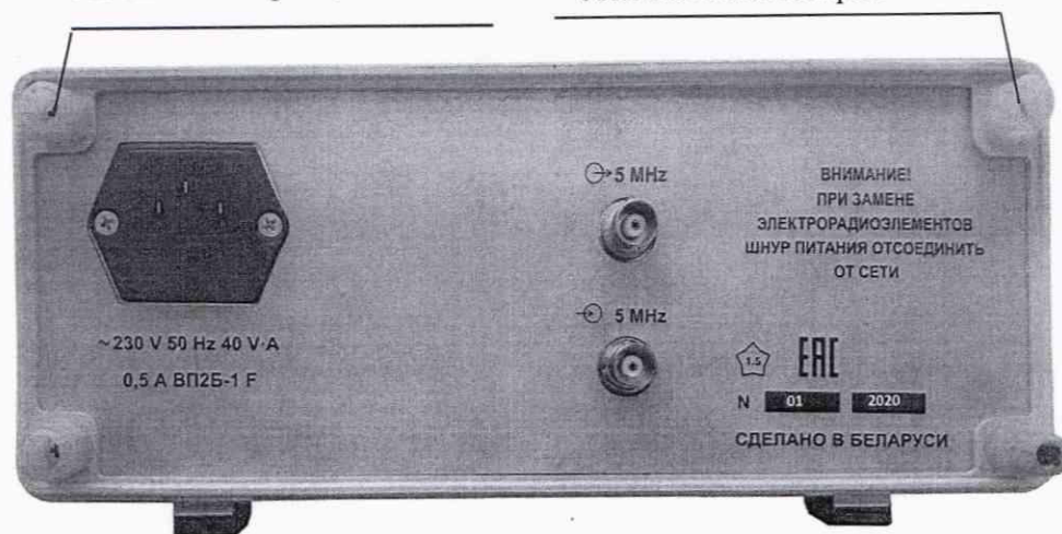
Рисунок 2.3 – Место пломбирования ОТК и нанесения оттиска знака поверки (вид частотомера сзади)
