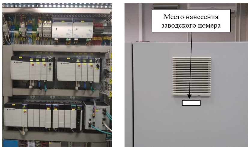
Рисунок 3 – Шкаф управления системы в сборе с указанием места расположения
