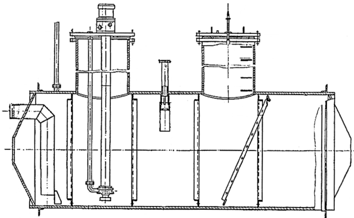
Рисунок 1 – Эскиз общего вида резервуара
