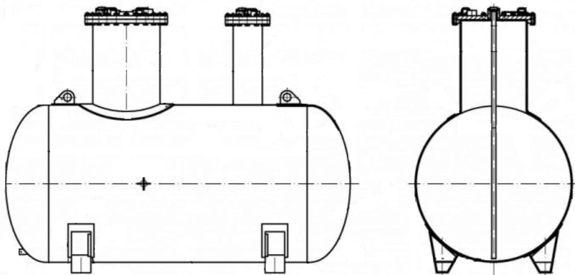
Рисунок 1 – Эскиз общего вида резервуара
