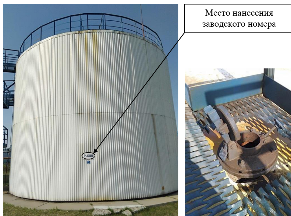
Р и с у н о к 2 – Общий вид резервуара с заводским номером Р-680 и его замерного люка
