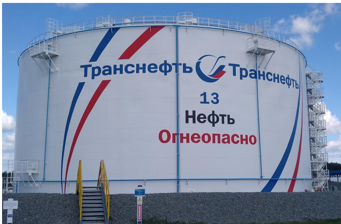
Рисунок 1 – Общий вид резервуара РВСП-20000 №13
