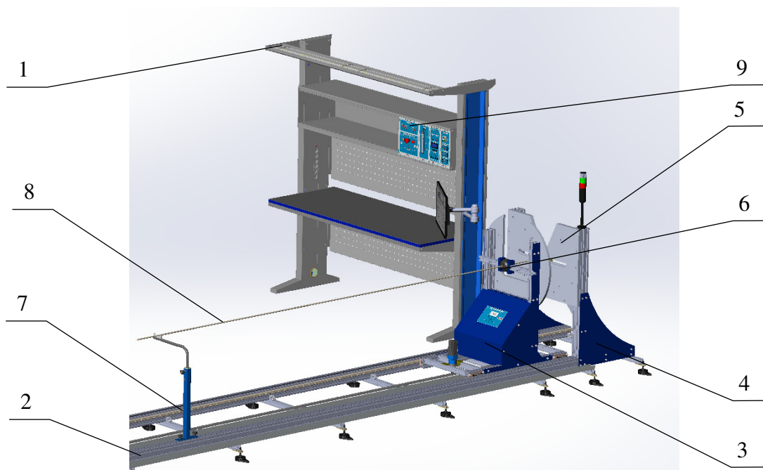
Р и с у н о к 3 – Общий вид установки при проверке поплавковых уровнемеров 1 – рабочее место оператора; 2 – линейная часть; 3 – подвижная часть; 4 – неподвижное основание; 5 – плита установочная; 6 – контактное приспособление; 7 – стойка поддержки; 8 – проверяемый прибор; 9 – шильд-панель (место нанесения заводского номера, даты изготовления и метрологических характеристик установки).
