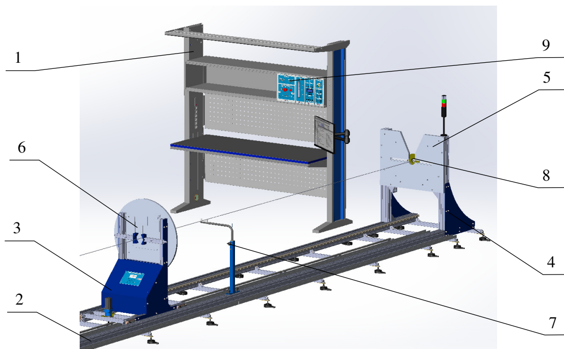
Р и с у н о к 1 – Общий вид установки при поверке волноводных уровнемеров 1 – рабочее место оператора; 2 – линейная часть; 3 – подвижная часть; 4 – неподвижное основание; 5 – плита установочная; 6 – контактное приспособление; 7 – стойка поддержки; 8 – поверяемый прибор; 9 – шильд-панель (место нанесения заводского номера, даты изготовления и метрологических характеристик установки).
