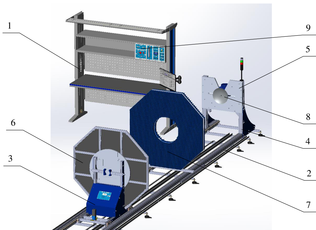
Р и с у н о к 2 – Общий вид установки при поверке радарных уровнемеров 1 – рабочее место оператора; 2 – линейная часть; 3 – подвижная часть; 4 – неподвижное основание; 5 – плита установочная; 6 – отражающая поверхность; 7 – экран для поглощения радиоволнового излучения и усечения луча; 8 – поверяемый прибор; 9 – шильд-панель (место нанесения заводского номера, даты изготовления и метрологических характеристик установки).
