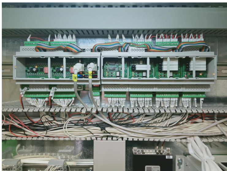
Рисунок 2 - Внешний вид контроллера в шкафу ПТК
