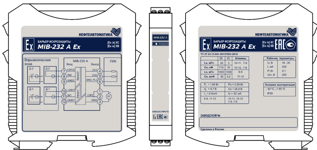
Рисунок 6 – Внешний вид исполнения MIB-232 A Ex
