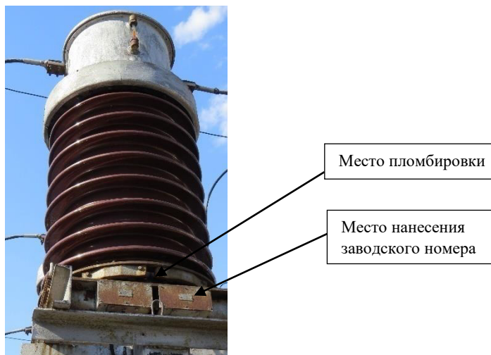
Рисунок 1 – Общий вид трансформатора тока ТФНД 110 с указанием места пломбировки от несанкционированного доступа, места нанесения заводского номера
