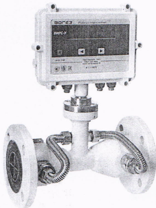
б) расходомер-счетчик DN25 – DN100 (фланцевое соединение исполнение С)
