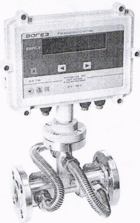
а) расходомер-счетчик DN15, DN20 фланцевое соединение (исполнение С (нержавеющая сталь))
