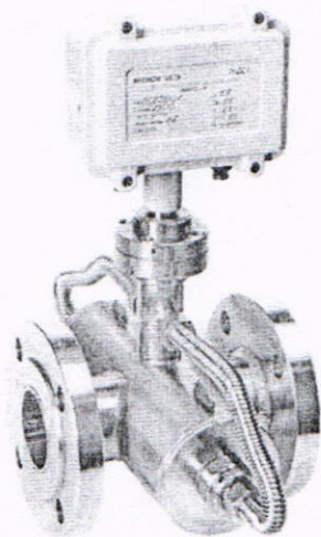
в) расходомер-счетчик DN50/1, DN50/2 (фланцевое соединение исполнение С)
