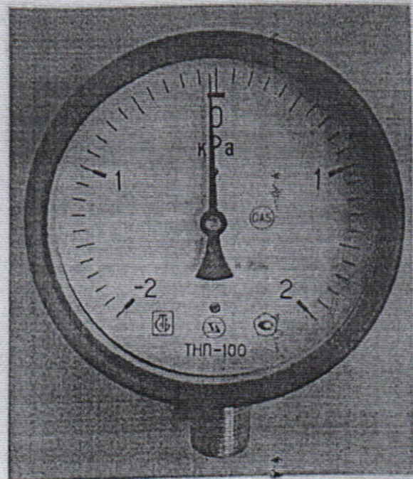
Тягонапоромер показывающий ТНП-100
