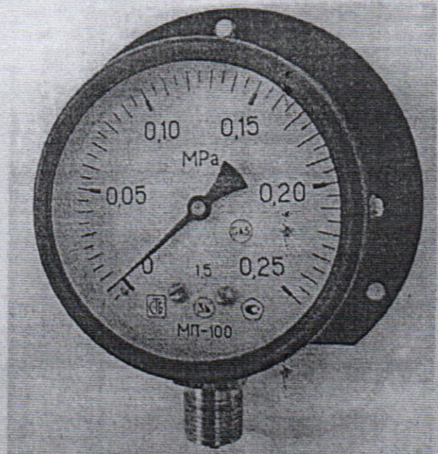
Манометр показывающий железнодорожного исполнения МП-100МД/Фз-Дм-Жд
