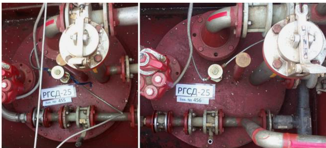
Рисунок 2 – Горловины и измерительные люки резервуаров РГСД-25 зав.№№ 455, 456
