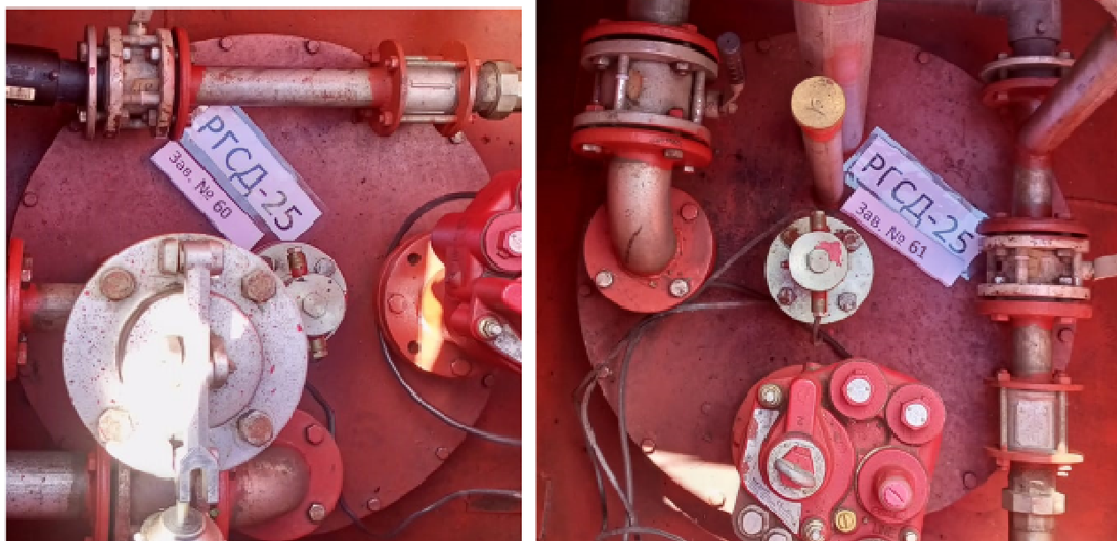
Рисунок 4 – Горловины и измерительные люки резервуаров РГСД-25 зав.№№ 60, 61
