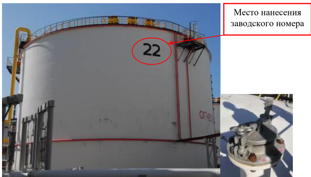
Рисунок 1 – Общий вид резервуара и замерного люка РВС-10000 зав.№ 22
