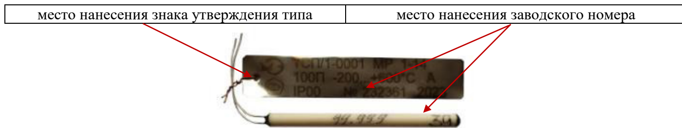
Рисунок 1 - Общий вид ТС модификации ТСП (ТСМ)/1-0001
