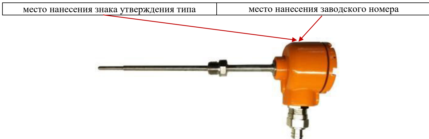
Рисунок 4 - Общий вид ТС модификации ТСП (ТСМ)/1-1187 с головкой А63 (конкретный вид защитной арматуры, узла крепления, и головки (соединителей или выводов) приведен в эксплуатационной документации)
