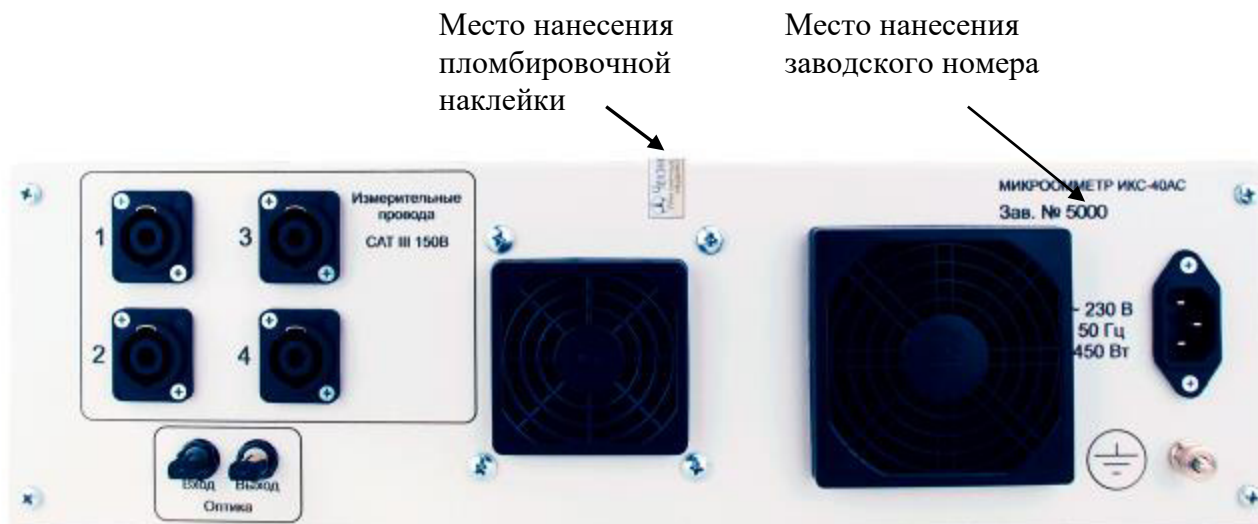
Рисунок 4 – Общий вид сзади микроамметров исполнения ИКС-40АС с местом нанесения пломбировочной наклейки и заводского номера
