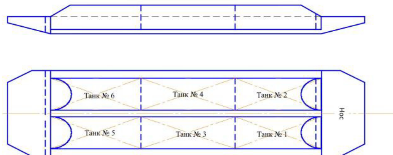
Рисунок 2 – Эскиз общего вида и расположения танков несамоходного наливного судна (баржи) «СТГН-12»
