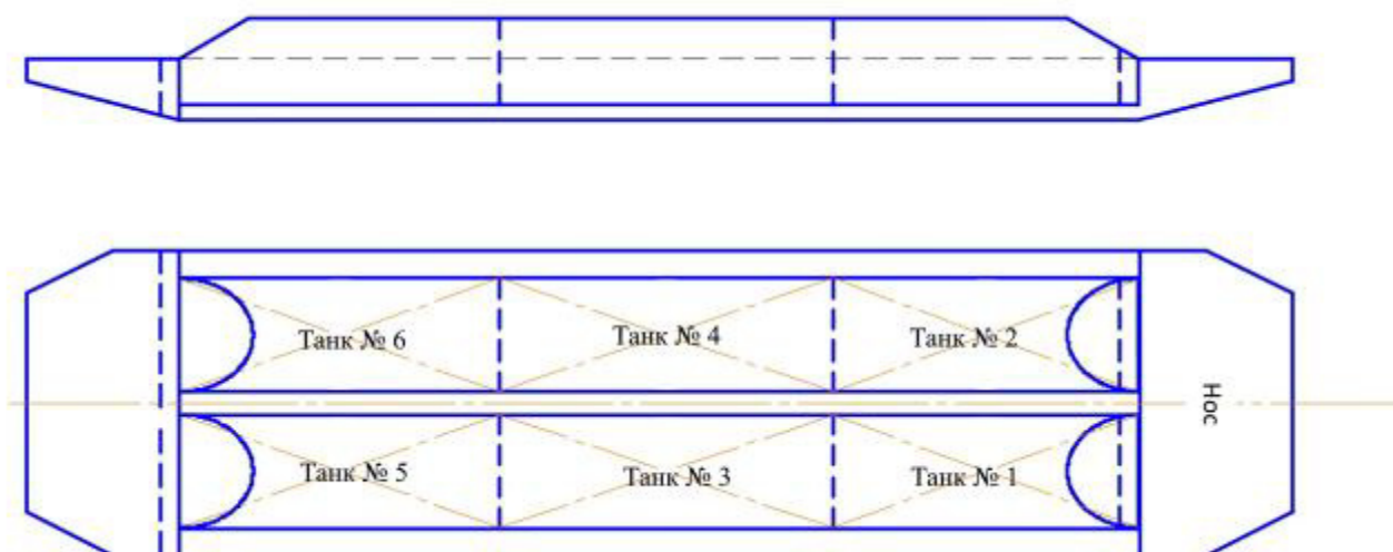
Рисунок 2 – Эскиз общего вида и расположения танков несамоходного наливного судна (баржи) «СТГН-15»
