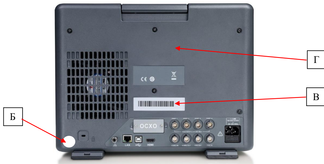
Рисунок 2 – Схема пломбировки от несанкционированного доступа (Б), место нанесения заводского номера (В) и место нанесения знака поверки (Г).
