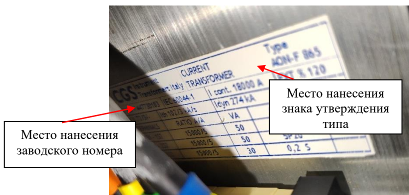
Рисунок 2 – Маркировочная табличка
