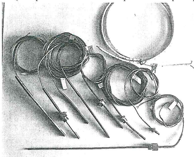
Рисунок 1.2 – Фотография общего вида преобразователей термоэлектрических ТХА(К)-1199, ТХК(Л)-1199, ТЖК(Л)-1199, ТНН(Н)-1199, ТПП(С)-1199, ТПП(Р)-1199, ТПР(В)-1199 в исполнениях без клеммной головки (изображение носит иллюстративный характер)
