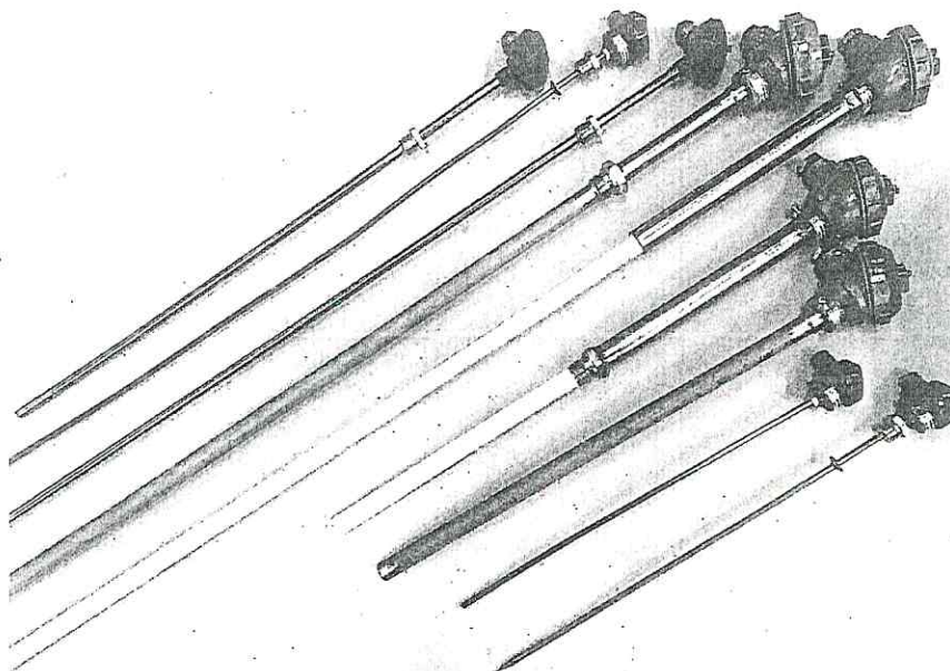
Рисунок 1.1 – Фотография общего вида преобразователей термоэлектрических ТХА(К)-1199, ТХК(Л)-1199, ТЖК(Л)-1199, ТНН(Н)-1199, ТПП(С)-1199, ТПП(Р)-1199, ТПР(В)-1199 в исполнениях с клеммной головкой (изображение носит иллюстративный характер)
