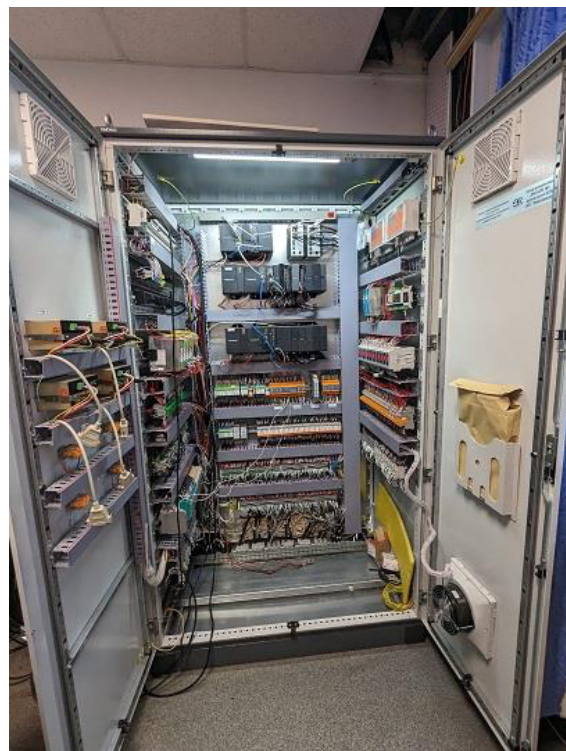
Рисунок 2 – Оборудование Комплекса
