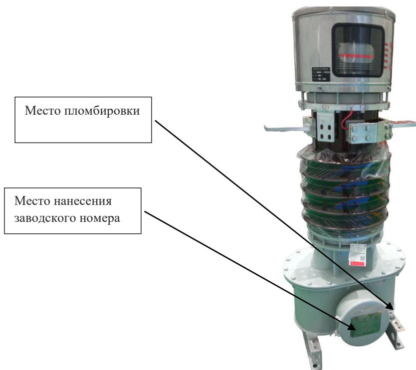
Рисунок 1 – Общий вид трансформатора тока LB6-35 с указанием места пломбировки от несанкционированного доступа, места нанесения заводского номера
