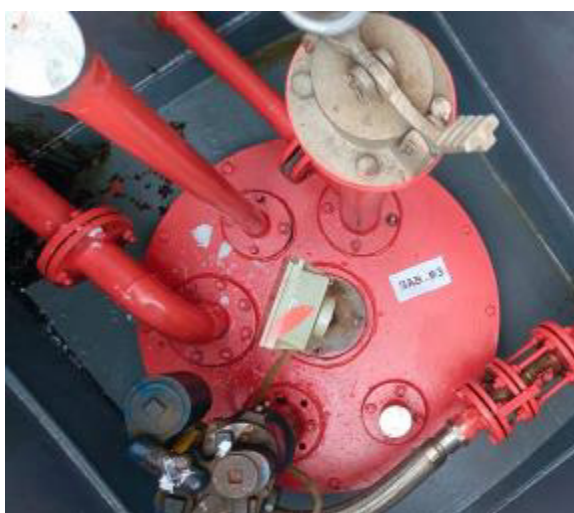
Рисунок 3 – Горловина резервуара РГС-20 зав.№ 3
