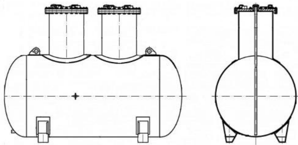
Рисунок 1 – Эскиз общего вида резервуаров
