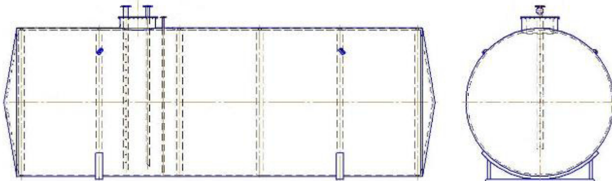
Рисунок 1 – Эскиз общего вида резервуаров
