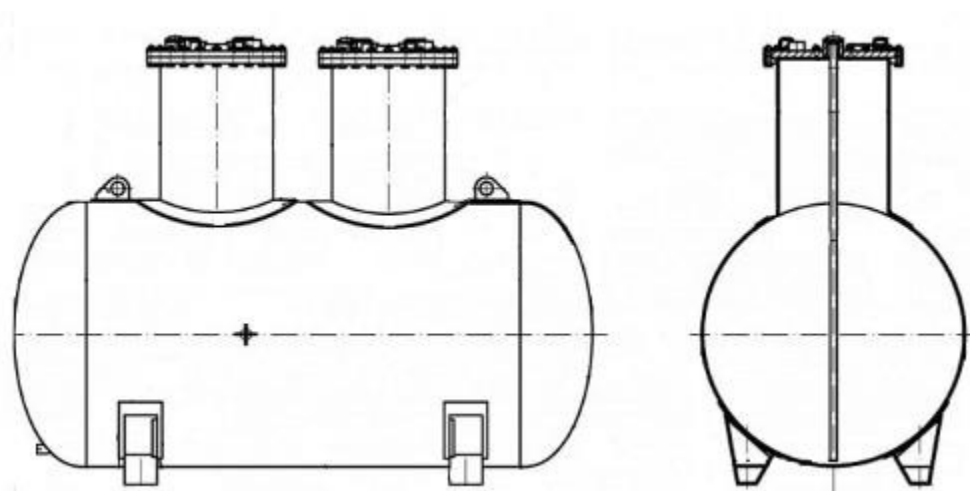
Рисунок 2 – Эскиз общего вида резервуаров РГС-50, РГС-60
