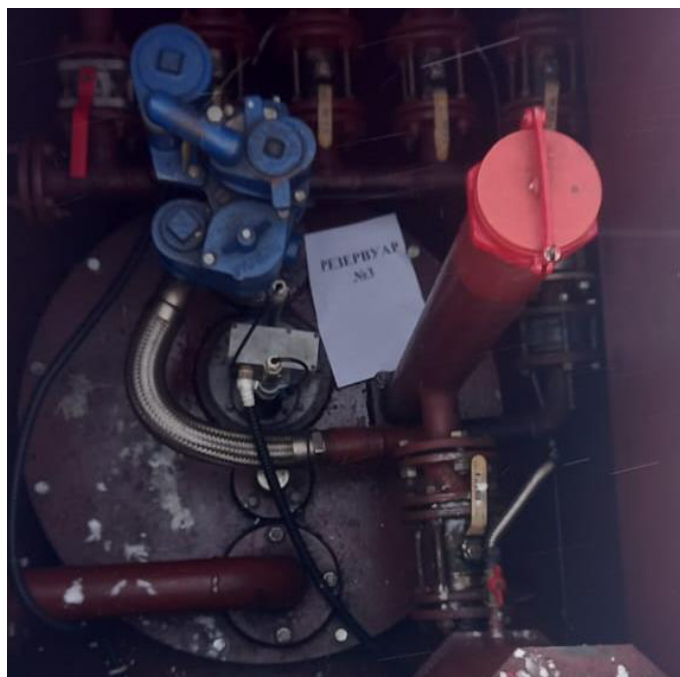
Рисунок 3 – Горловина резервуара РГС-63 зав.№ 3
