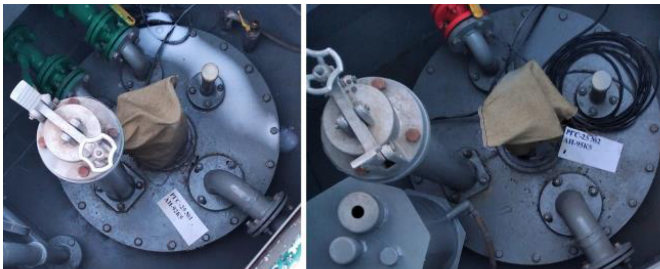
Рисунок 2 – Горловины резервуаров PFC-25 зав.№№ 1, 2
