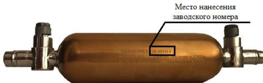
Рисунок 1 – Общий вид пикнометра с указанием места нанесения заводского номера
