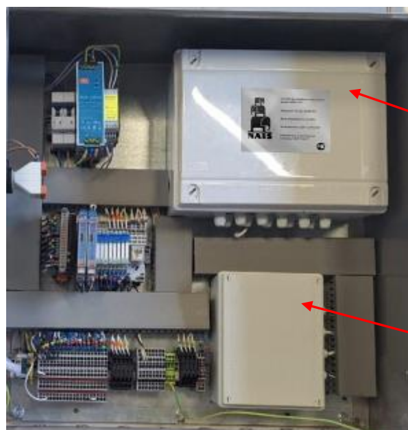
шкаф управления
