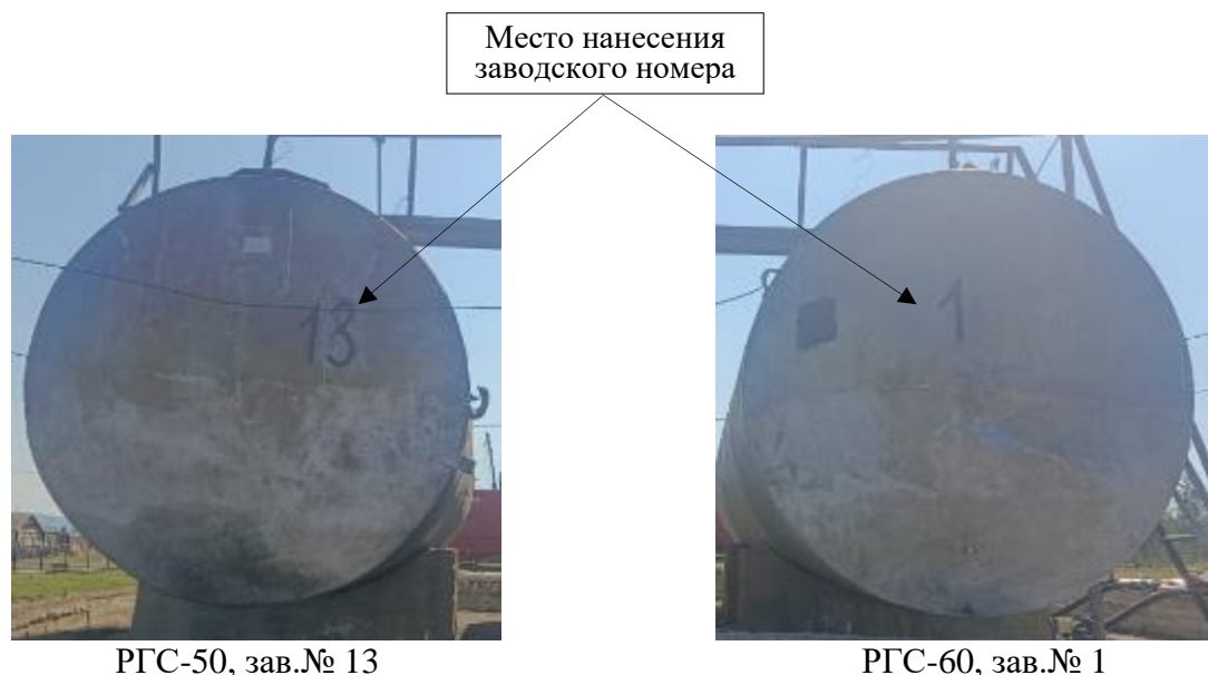
Рисунок 1 – Общий вид резервуаров
