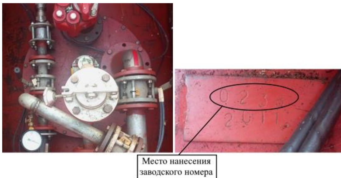
Рисунок 9 – Горловина и измерительный люк резервуара РГП 25-1-2(0,85)-О-У зав.№ 0238
