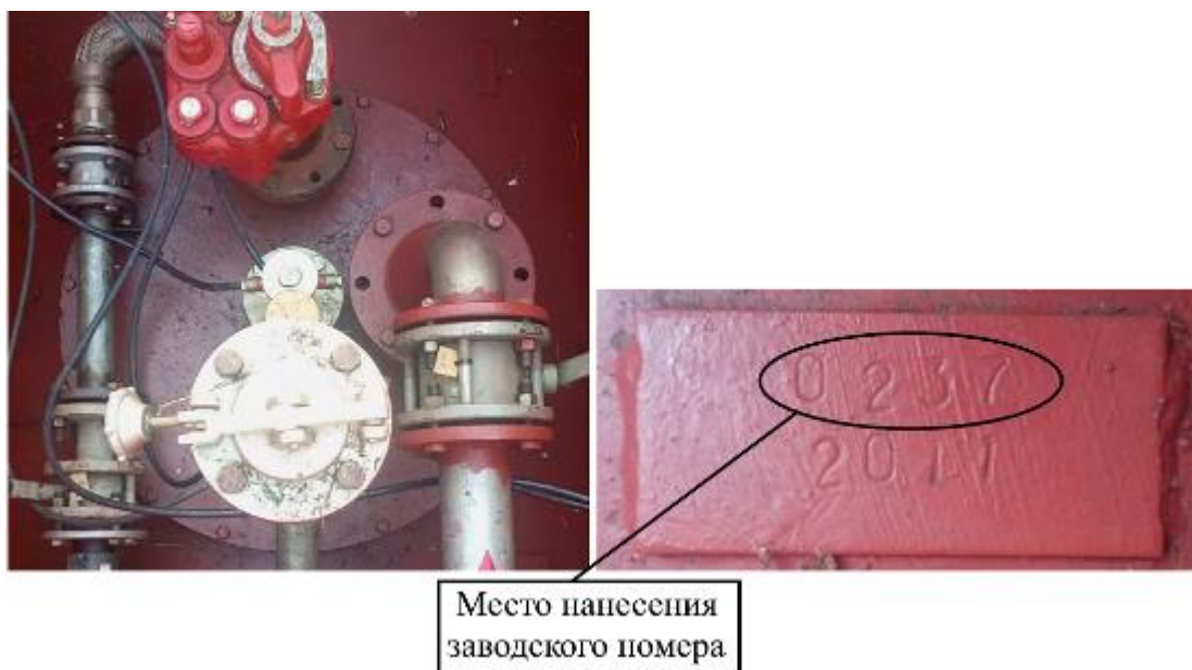
Рисунок 7 – Горловина и измерительный люк резервуара РГП 25-1-2(0,85)-О-У зав.№ 0237
