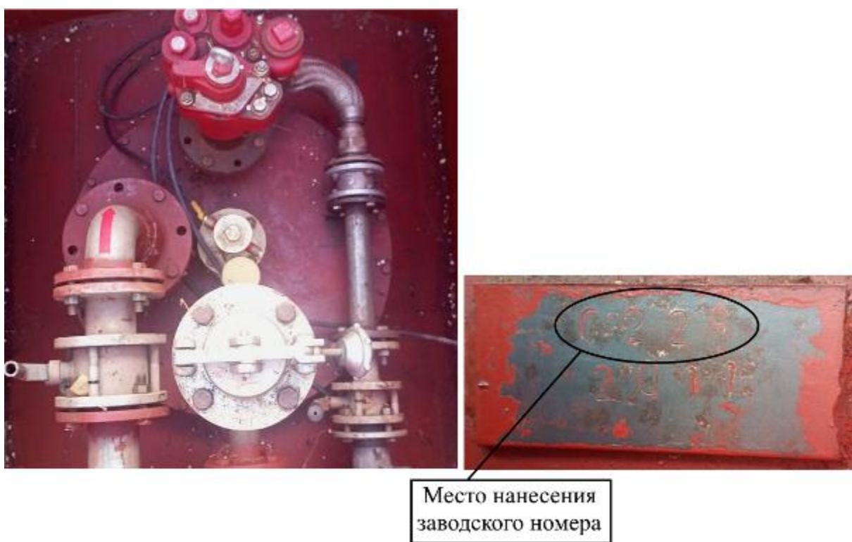
Рисунок 2 – Горловина и измерительный люк резервуара РГП 25-1-2(0,85)-О-У зав.№ 0228
