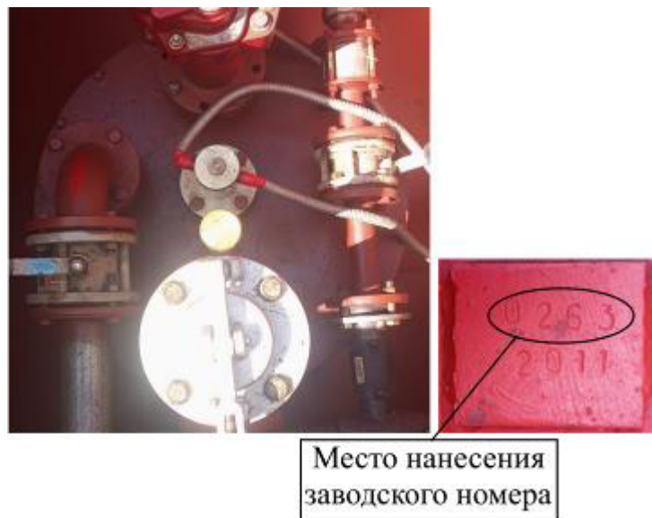
Рисунок 7 – Горловина и измерительный люк резервуара РГП 25-1-2(0,85)-О-У зав.№ 0263
