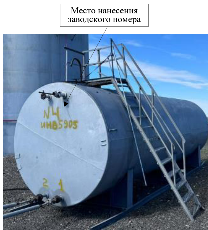
Рисунок 1 – Общий вид резервуара, зав. № 4
