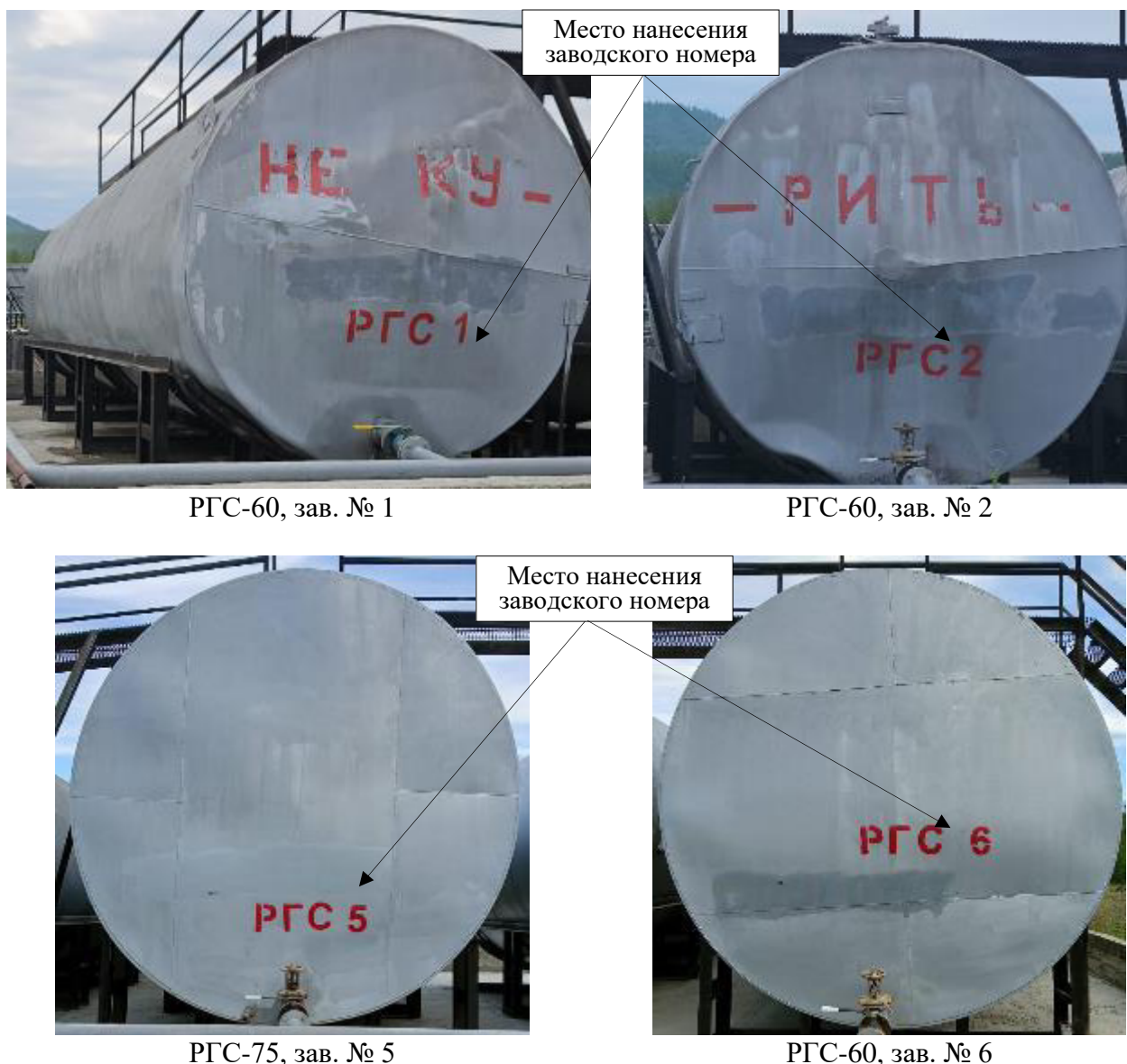
Рисунок 1 – Общий вид резервуаров
