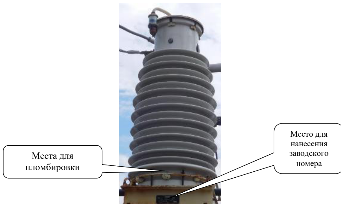
Рисунок 1 – Общий вид трансформаторов напряжения с указанием мест пломбировки, места нанесения заводского номера
