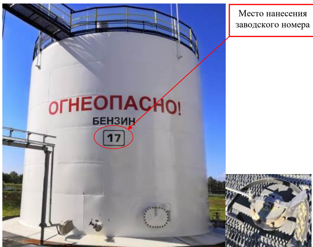
Рисунок 2 – Общий вид резервуара и замерного люка РВС-700 зав. № 17
