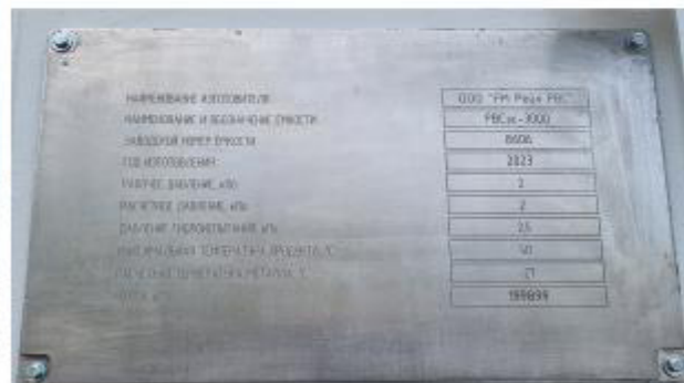
Рисунок 2 – Общий вид маркировочной таблички и резервуара РВСзс-3000 зав.№ 8606
