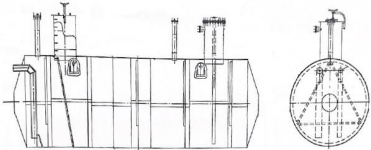
Рисунок 1 – Эскиз общего вида резервуаров
