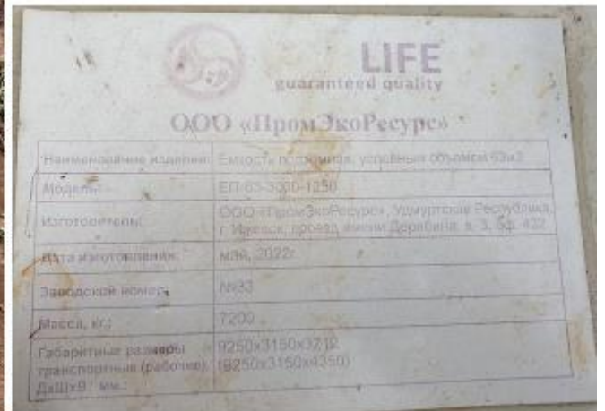
Рисунок 2 – Общий вид маркировочной таблички и горловины резервуара ЕП-63-3000-1250 зав.№ 33
